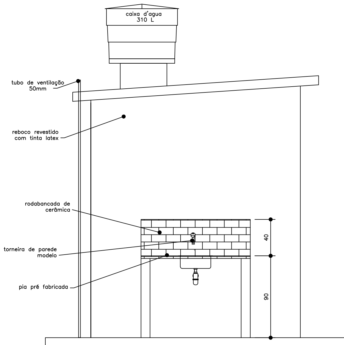
ELEVAÇÃO LATERAL ESC. 1/25
