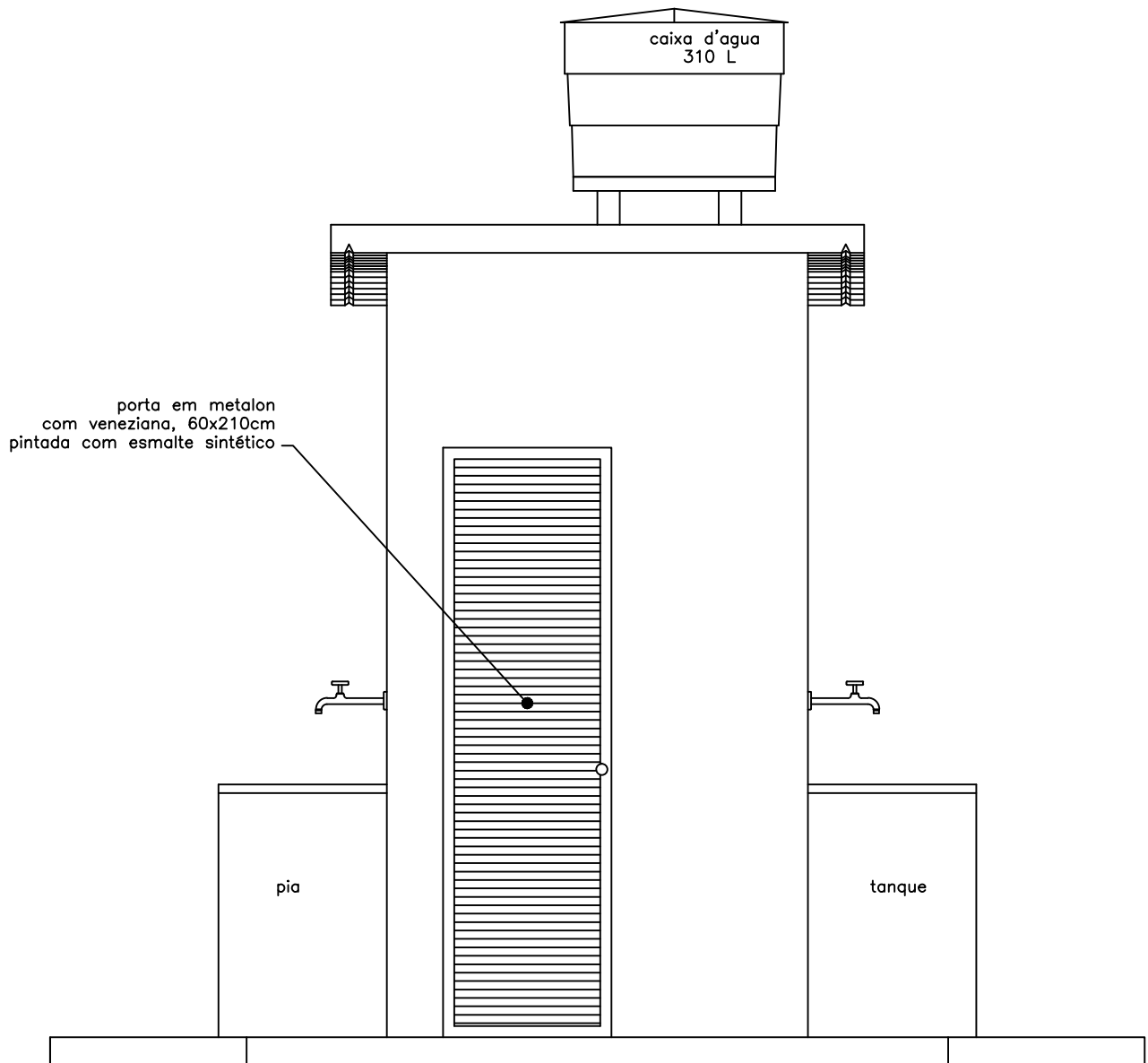
ELEVAÇÃO FRONTAL ESC. 1/25
